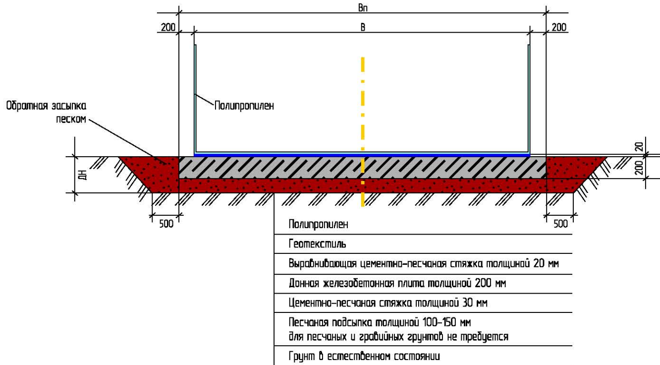
Рисунок №2. Схема устройства бассейна из полипропилена на поверхности земли.
