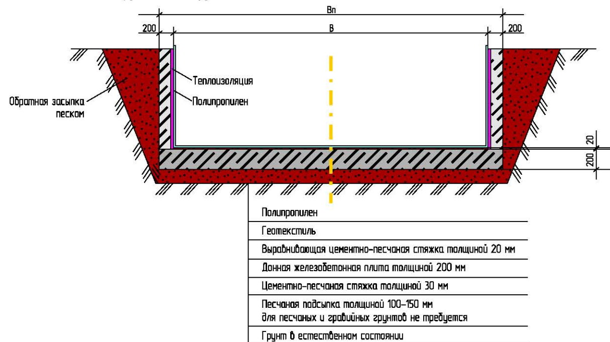
Рисунок №3. Схема устройства бассейна из полипропилена частично либо полностью погруженного в грунт.
